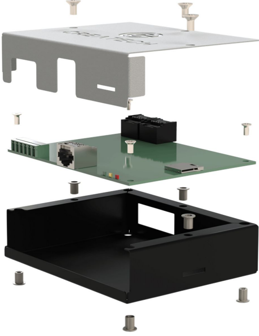
Demontaj
